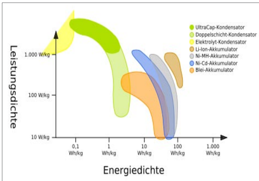
Abbildung 3-1: Vergleich von Leistungs- und Energiedichte von einigen Energiespeichern (MIT 2007)
