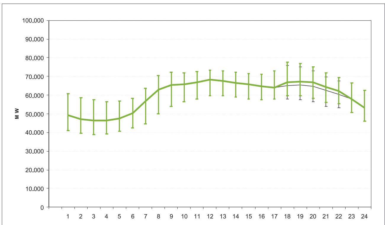
Abbildung 5-7: Entwicklung des Tageslastgangs (Mittel-, Höchst- und Tiefstwerte) am Mittwoch bei einer ungesteuerten Aufladung über 5 Stunden von 1 Mio. netz-elektrischer Fahrzeuge werktäglich um 18 Uhr
