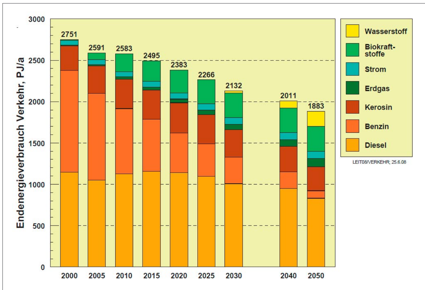
Abbildung 4-1: Energieeffizienz im Verkehr im Leitszenario 2006 nach Kraftstoffarten (Nitsch 2008)
