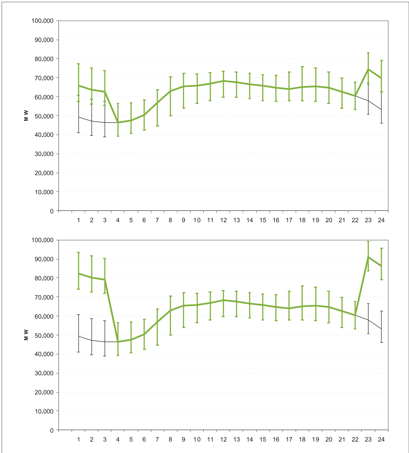
Abbildung 5-11: Entwicklung des Tageslastgangs (Mittel-, Höchst- und Tiefstwerte) am Mittwoch bei einer gesteuerten Aufladung über 5 Stunden von 10 Mio. und 20 Mio. netz-elektrischer Fahrzeuge kalendertäglich um 23 Uhr
