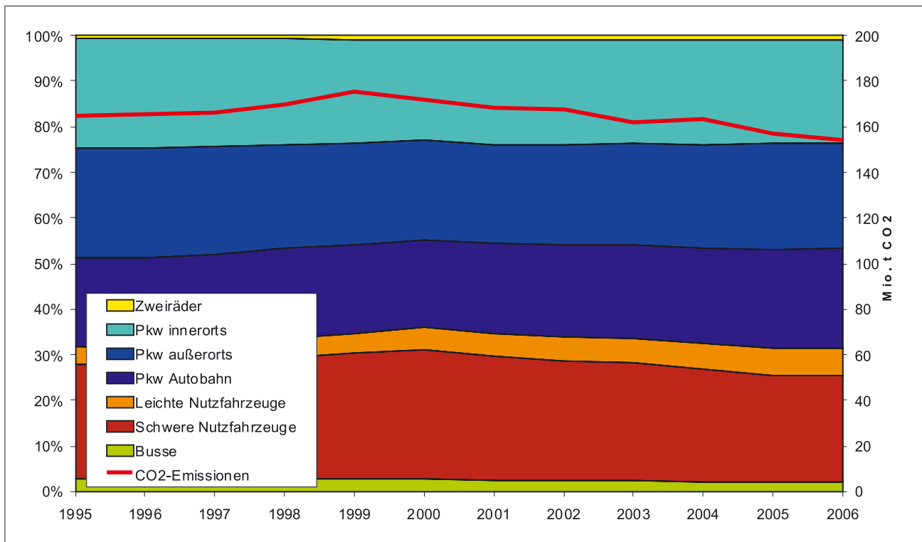
Abbildung 5-1: CO 2 -Emissionen des Straßenverkehrs in Deutschland, absolut und Struktur nach Verkehrsträgern (Umweltbundesamt)
