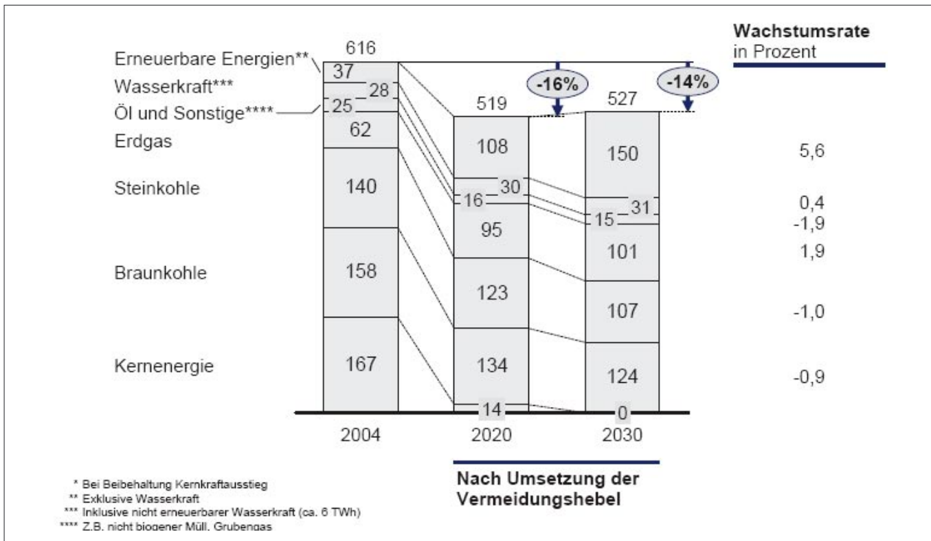
Abbildung 4-2: Bruttostromerzeugung nach Umsetzung der Vermeidungshebel – Deutschland 2004 – 2030*(McKinsey 2007)
