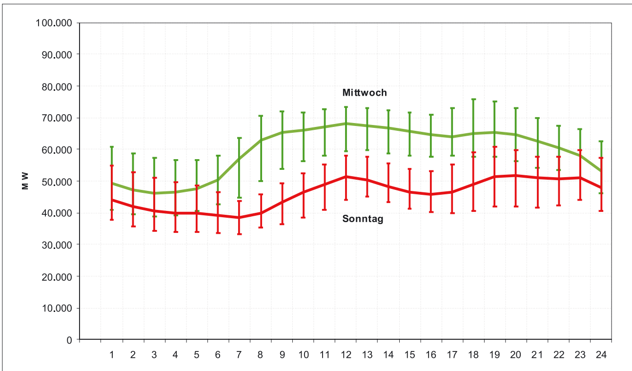
Abbildung 5-5: Durchschnittlicher Tageslastgang, Höchst- und Tiefstlast im deutschen Verbundsystem, Mittwoch und Sonntag (UCTE)
