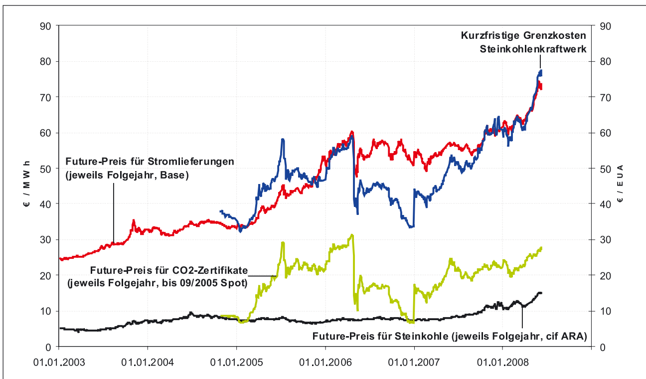
Abbildung 5-3: Preisverlauf der Future-Kontrakte für Strom, Steinkohle und CO 2 -Zertifikate sowie die kurzfristigen Grenzkosten eines hypothetischen Grenzkraftwerks nach Matthes/Ziesing (2008)
