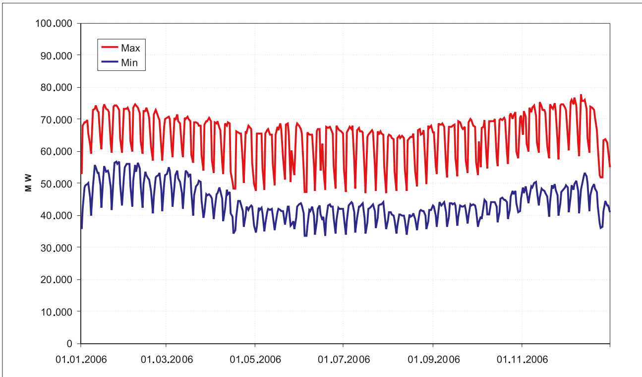
Abbildung 5-4: Tägliche Höchst- und Tiefstlast im deutschen Verbundsystem im Jahr 2006 (UCTE)
