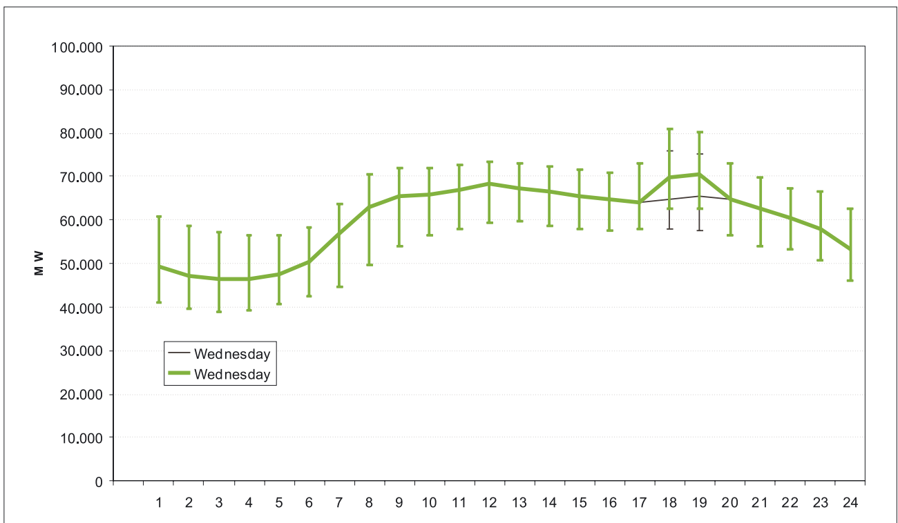
Abbildung 5-9: Entwicklung des Tageslastgangs (Mittel-, Höchst- und Tiefstwerte) am Mittwoch bei einer ungesteuerten Aufladung über 2 Stunden von 1 Mio. netz-elektrischer Fahrzeuge werktäglich um 18 Uhr
