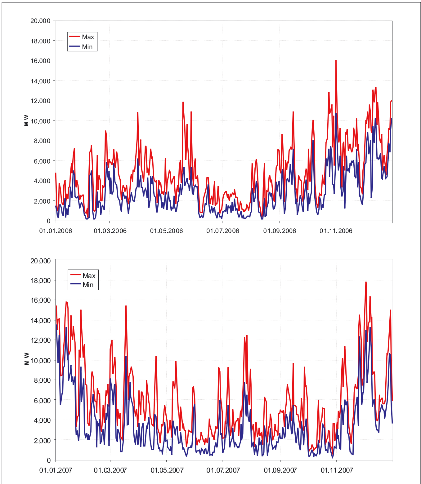
Abbildung 5-6: Höchst- und Tiefwerte der kalendertäglichen Windenergieeinspeisung für das Jahr 2006 und 2007 (Verbundnetzbetreiber)
