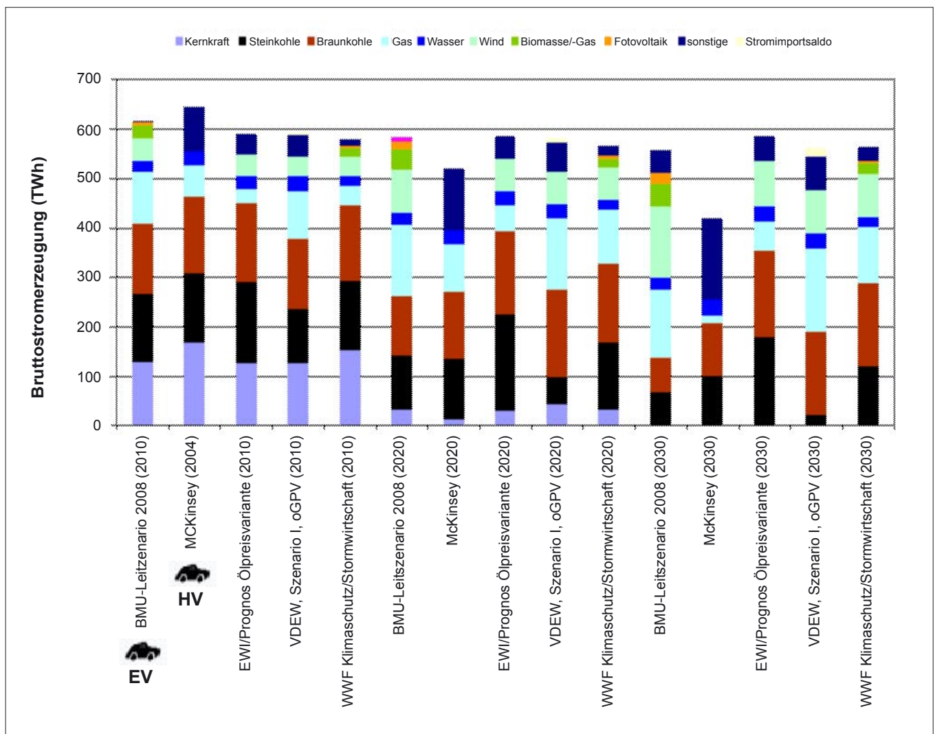
Abbildung 4-4: Gegenüberstellung der Kraftwerksparkentwicklung in verschiedenen Szenarien für die Jahre 2010, 2020 und 2030
