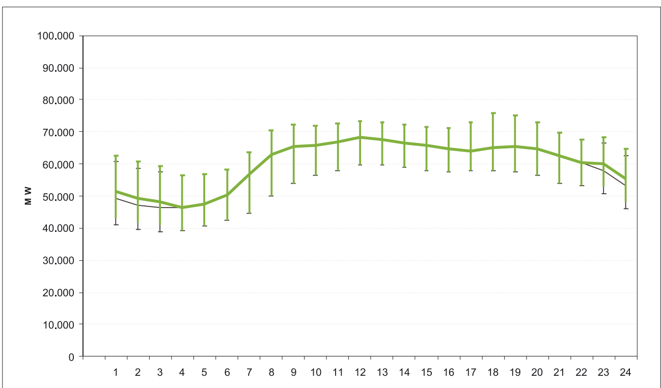
Abbildung 5-10: Entwicklung des Tageslastgangs (Mittel-, Höchst- und Tiefstwerte) am Mittwoch bei einer gesteuerten Aufladung über 5 Stunden von 1 Mio. netzelektrischer Fahrzeuge werktäglich um 23 Uhr
