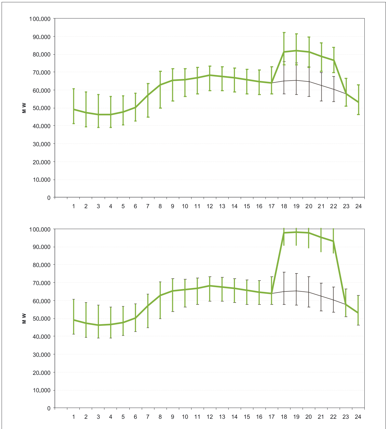
Abbildung 5-8: Entwicklung des Tageslastgangs (Mittel-, Höchst- und Tiefstwerte) am Mittwoch bei einer ungesteuerten Aufladung über 5 Stunden von 10 Mio. und 20 Mio. netz-elektrischer Fahrzeuge kalendertäglich um 18 Uhr (Extremszenario)
