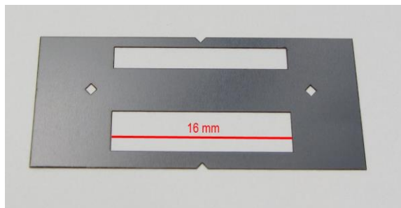
Kontaktschichtmaske aus Metallfolie
