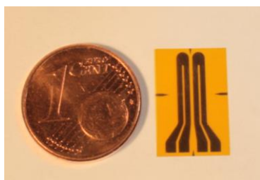
U-Struktur für Biegebalken
