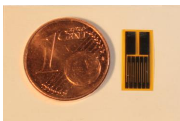
Mäanderförmige DMS-Struktur
