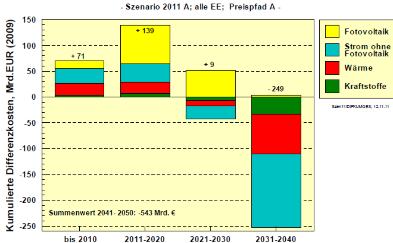
Abbildung 19: Kumulierte systemanalytische Differenzkosten der gesamten Energiebereitstellung aus EE im Szenario 2011 A für 10-Jahres-Abschnitte und Preisfad A
